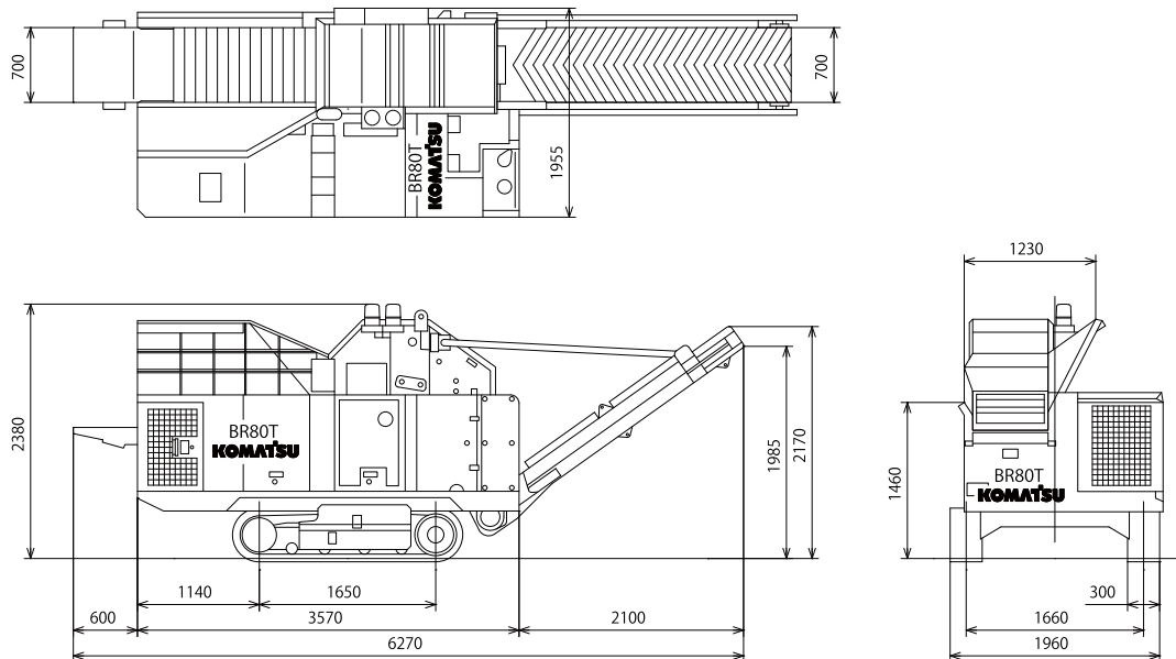
BR80T 寸法図 (単位: mm)
