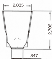
DTS65 寸法図 (単位: mm)
