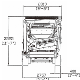
TRM622 寸法図 (単位: mm)
